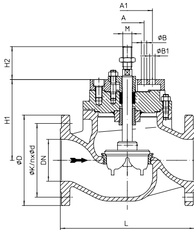
Fig. 470...90 DN200 / NPS 8" (z.B.: DP34, PREMIO 5-25kN)
